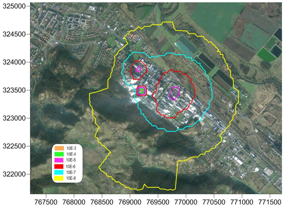
A BorsodChem Zrt. aktuális összesített egyéni halálózási kockázata
