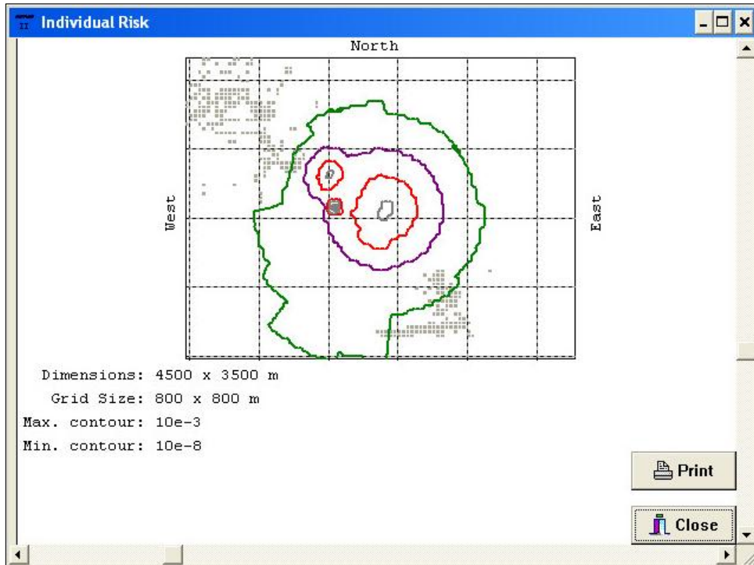
A BorsodChem Zrt. mérgezésre és robbanásra megadott összesített egyéni halálózási görbéinek összege SAVEII kockázatelemző szoftver modellterében
