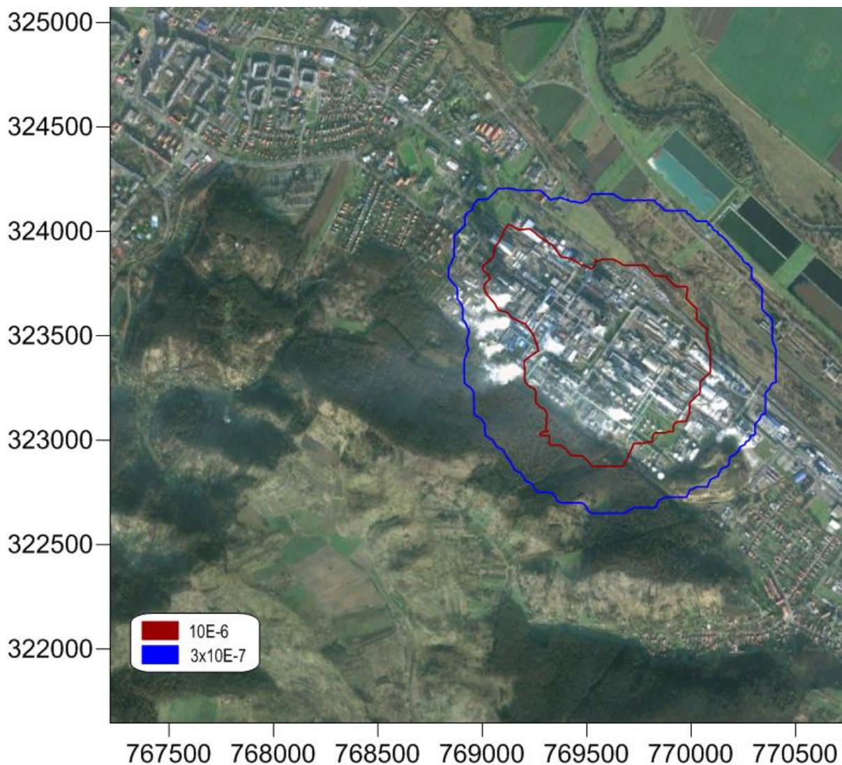
A BorsodChem Zrt. tevékenységéből származó aktualizált sérülés egyéni kockázati görbéi
